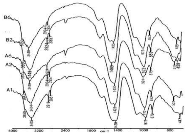
图4 气凝胶不同掺量时发泡混凝土FT-IR图谱。
