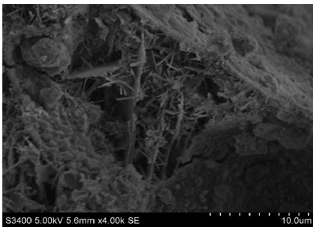
图6 掺加0.05%纤维素醚后的发泡混凝土SEM图。
