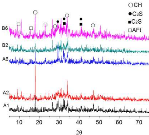
图3 气凝胶不同掺量时发泡混凝土XRD图谱。
