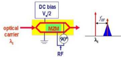
Fig. 2. OSSB+C signal generation using DEMZM.
