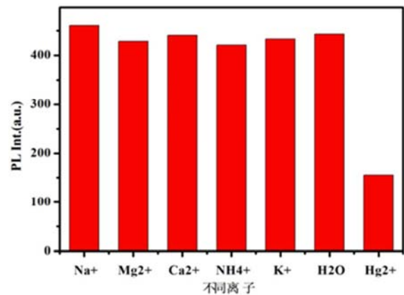
图5 不同离子条件下溶液荧光强度对比。
