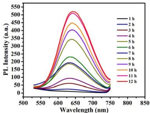
图3 反应时间对所制备的Au-BSANCs荧光强度的影响。
