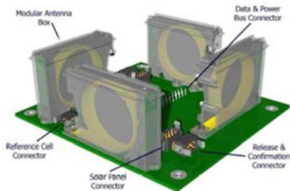
图1 Delfi-C3卫星测控天线。
