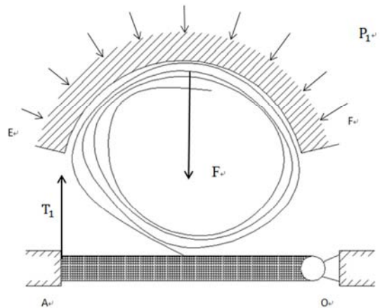
图4 摇臂式结构展开前示意图。
