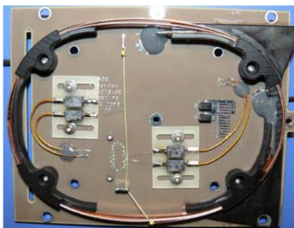
图2 Swisscube卫星天线。
