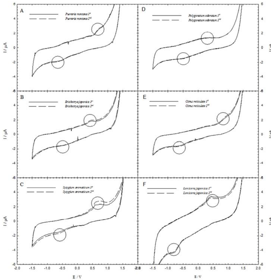
圖1 各種中草藥在未微生物脫色前之循環伏安比較圖譜(圈處代表可能具有氧化還原活性之峰值位置)。
