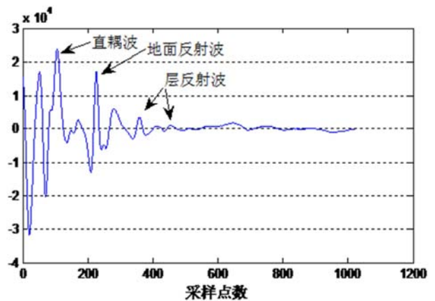
图2 雷达实测反射信号。
