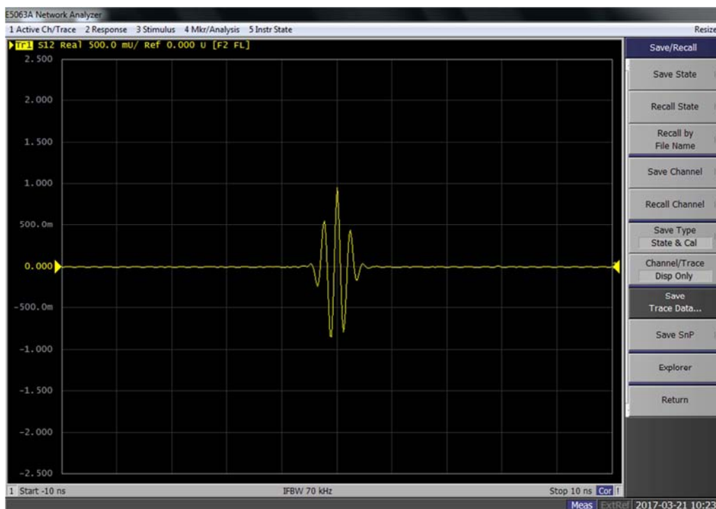
图6 矢量网络分析仪发射波形。
