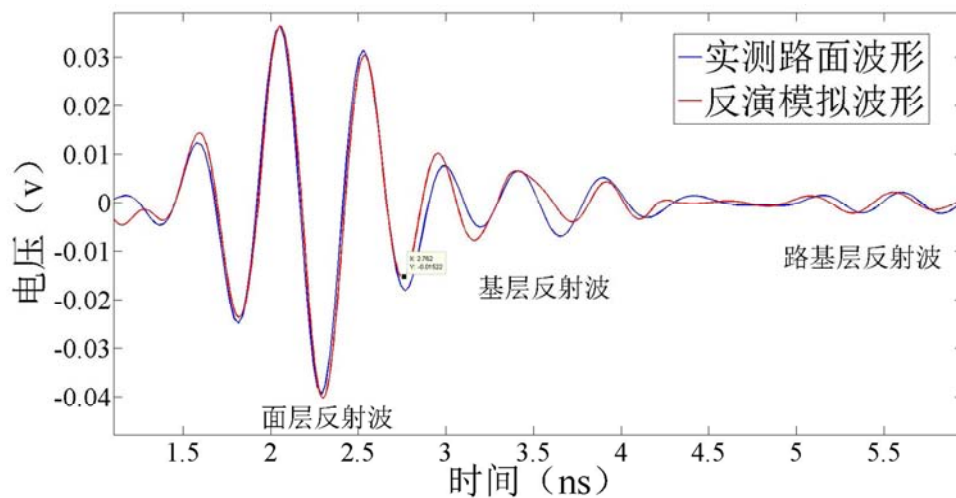
图12 实际路面反演结果。
