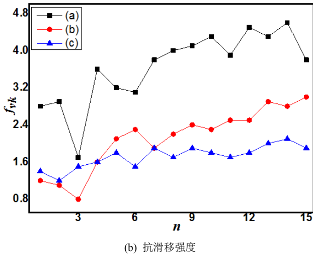
图3 试验结果分析图。
