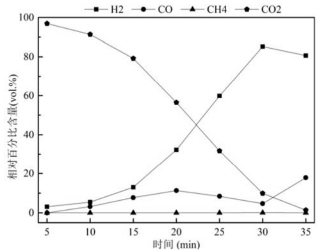
(d) 焙烧温度900°C
