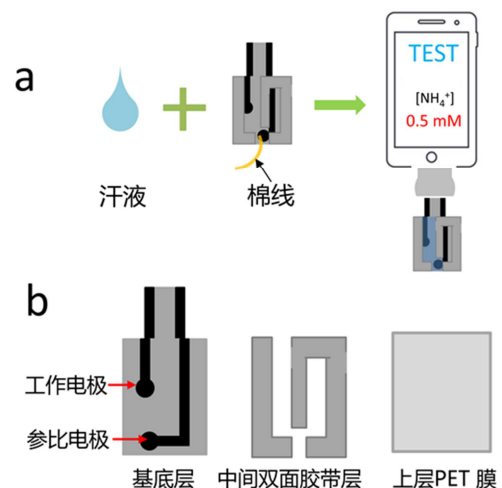
图1 (a) 基于智能手机的传感器用于汗液铵离子的检测; (b) 三层的汗液铵检测传感器。第一层是制备的电极衬底, 第二层是双面胶带和棉线, 第三层是一个亲水层, 以方便样品的毛细作用。
