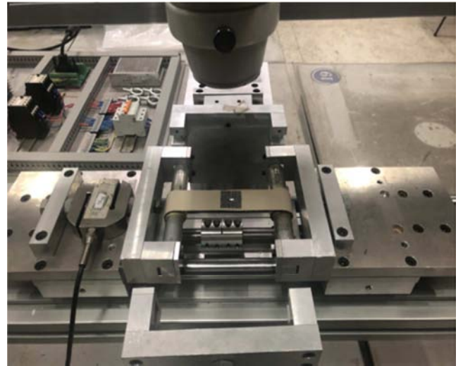
图1 双轴万能拉伸试验机。
