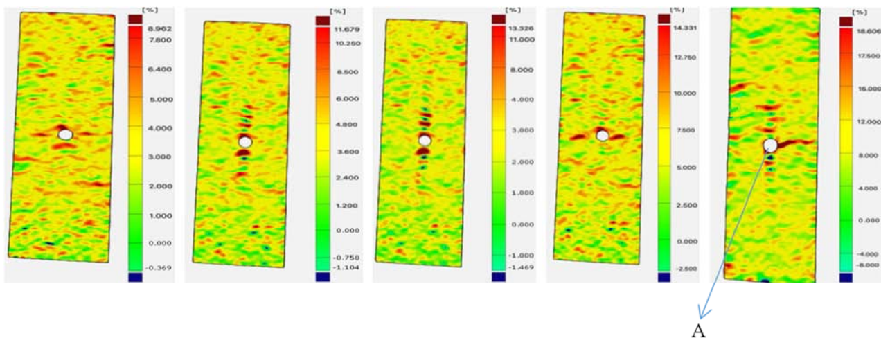
(a)中心2mm孔应变云图演变
