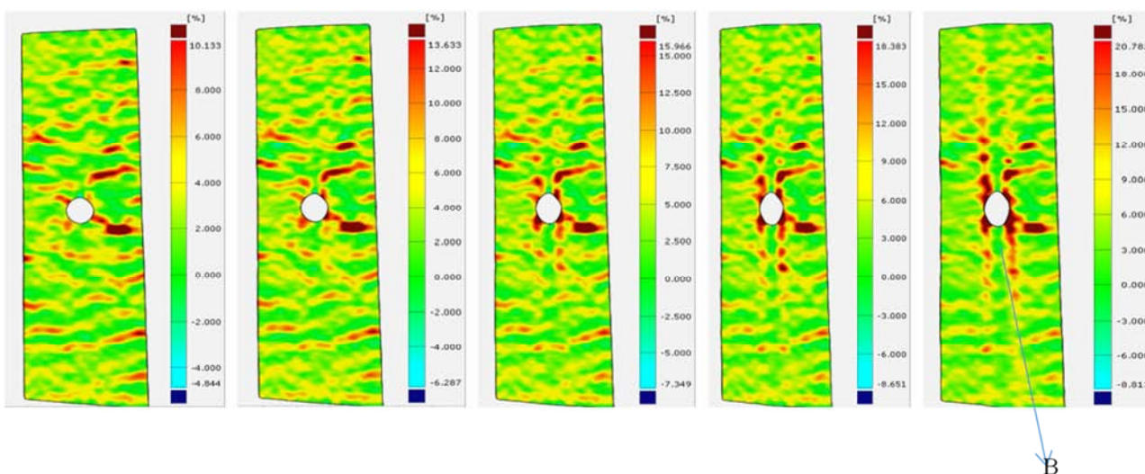
(b)中心4mm孔应变云图演变
