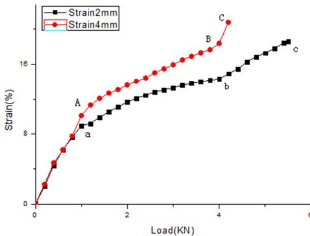
图6 膜材双向拉伸下最大应变场指标演化图。
