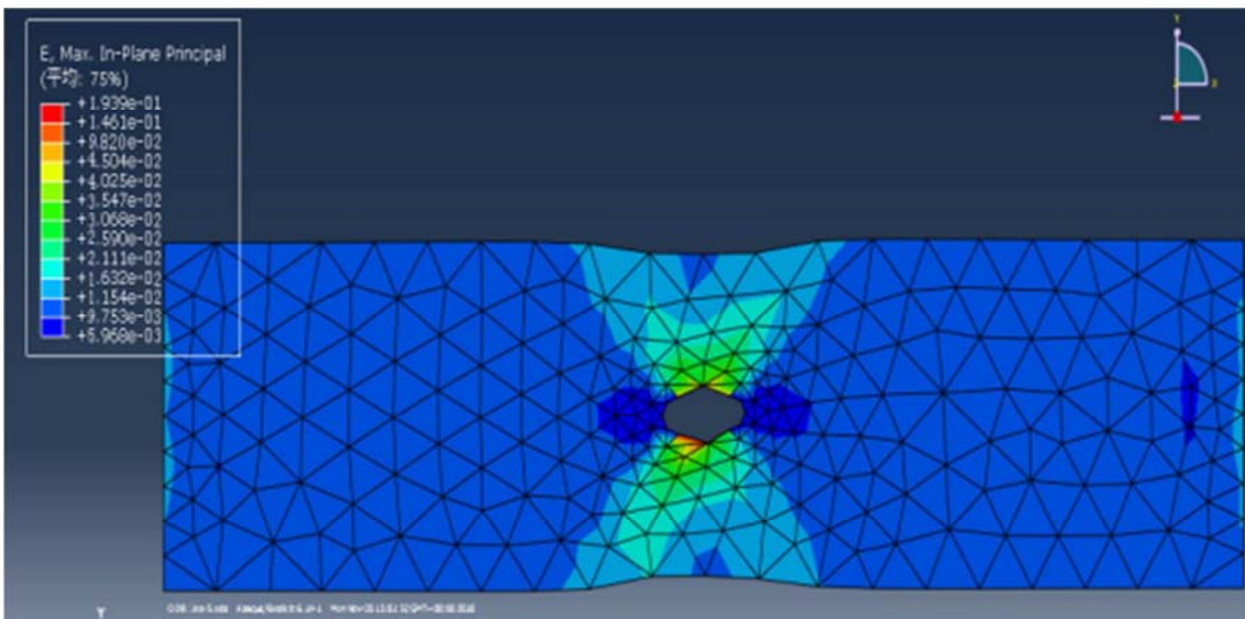
(a)2mm中心孔模型
