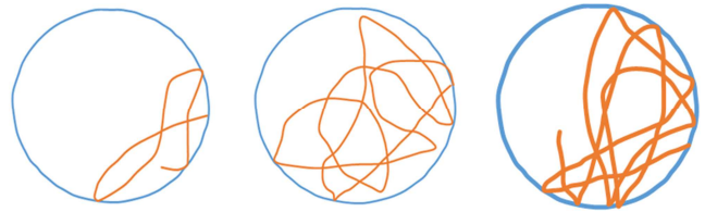
图5 30、60和90RPM转速下，井深3800m处的钻柱中心运动轨迹图。
