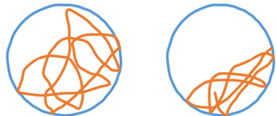
图6 6 \times 10^4 \text{N} 和 10 \times 10^4 \text{N} 钻压下，井深3800米处的钻柱中心运动轨迹图。
