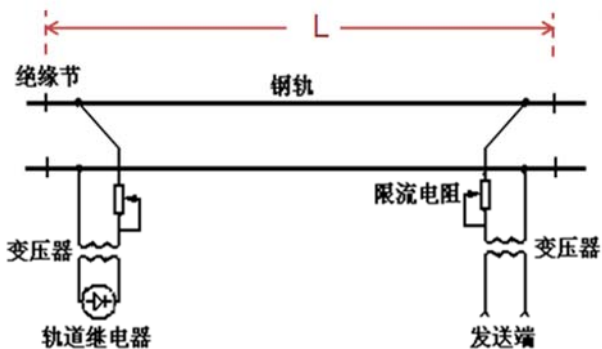
图5 实验轨道电路模型示意图。
