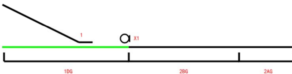
图10 办理直向进路区段图。
