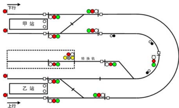
图3 实验线路图。
