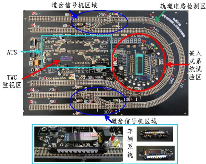
图1 轨道交通信号与控制教学实验系统实物图。
