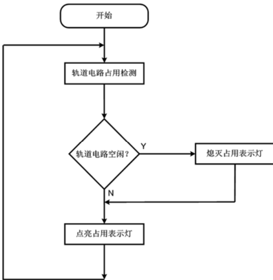
图9 轨道电路检测流程图。
